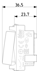
Vista ingombri
