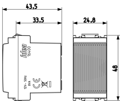
Vista ingombri
